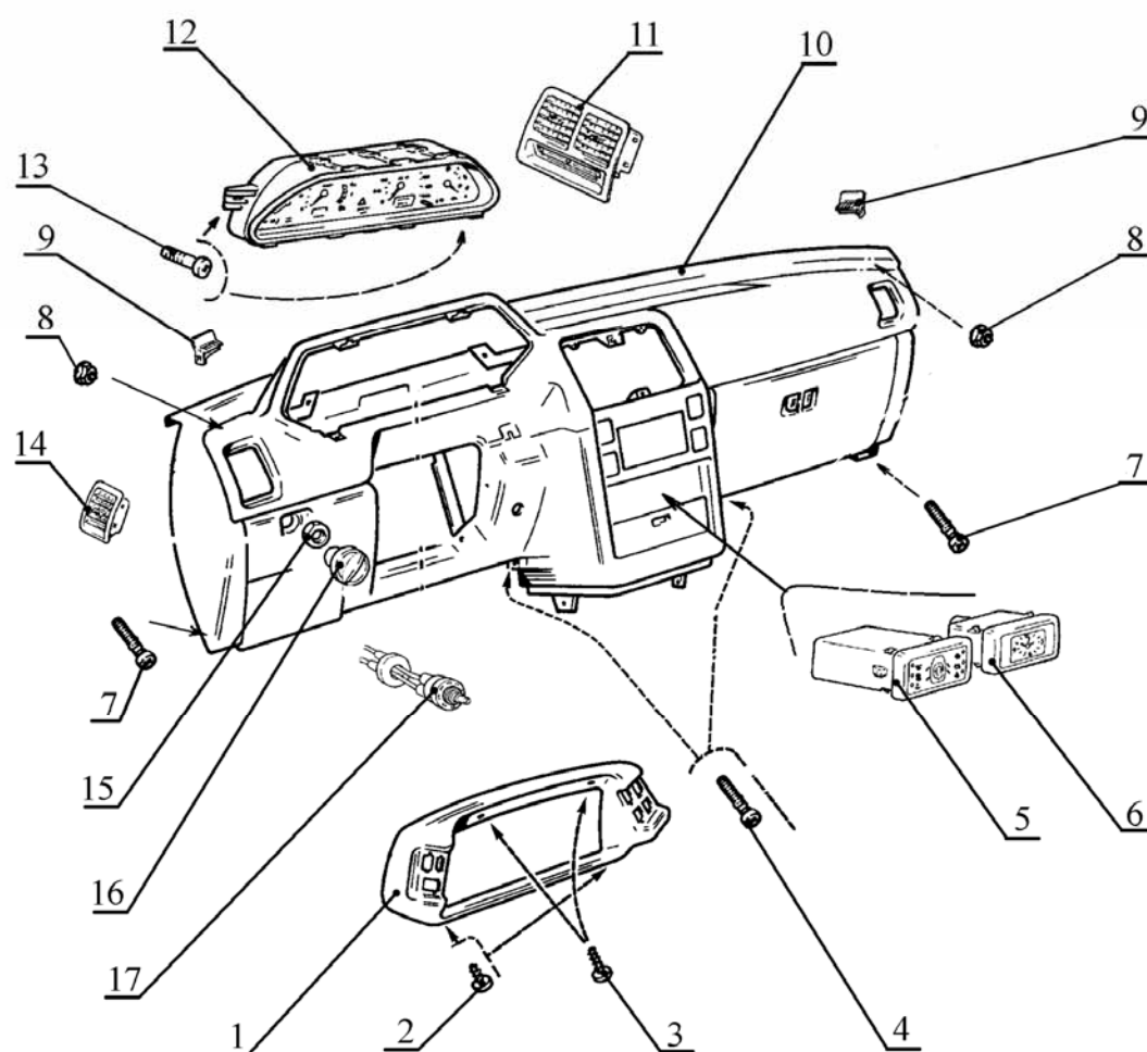
Рисунок 3 – Панель приборов 2110-5325010:
