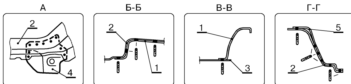
Рис.10. Детали арки ВАЗ-2111 заднего колеса наружной с угловой панелью боковины в сборе правой/левой. Номера и наименования деталей, количество сварочных точек приведены в таблице 10. Места, указанные стрелками, проварить сплошным швом длиной 40 мм (см. поз.2 табл.10).
