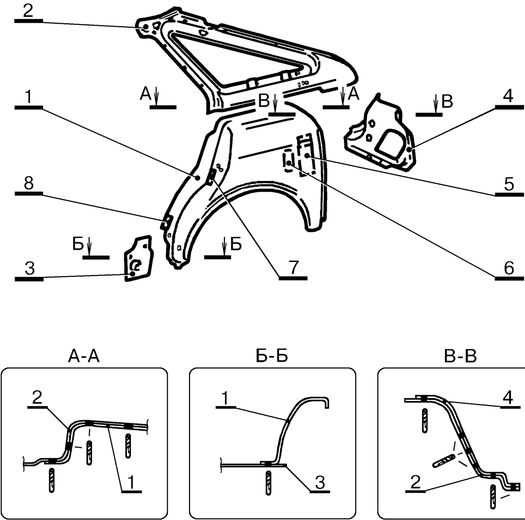
Рис.12. Детали арки ВАЗ-2112 заднего колеса наружной с угловой панелью боковины в сборе правой/левой. Номера и наименования деталей, количество сварочных точек приведены в таблице 12.
