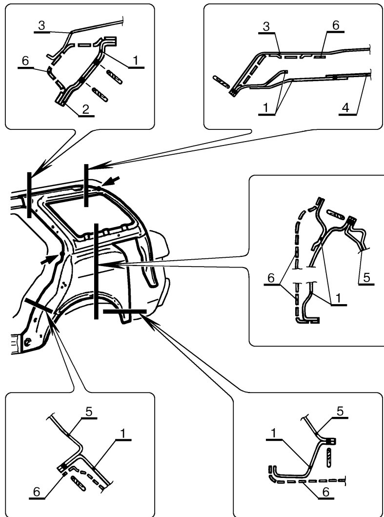
Рис.9. Соединение арки 2111-5401170/171 заднего колеса наружной с угловой панелью боковины в сборе правой/левой с сопрягаемыми деталями (при снятой двери задка, заднем крыле и желобке заднего крыла). Места, указанные стрелками, проварить сплошным швом длиной 40 мм (см. поз.3 и 5 табл.9).
