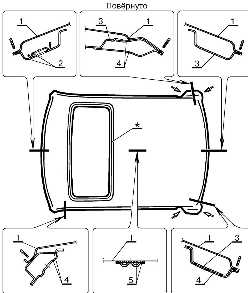
Рис.3. Соединение панели крыши в сборе ВАЗ-2110 с сопрягаемыми деталями (при снятых дверях). Места, указанные стрелками, проварить сплошным швом длиной 20 мм (см. поз.4 табл. 3)
