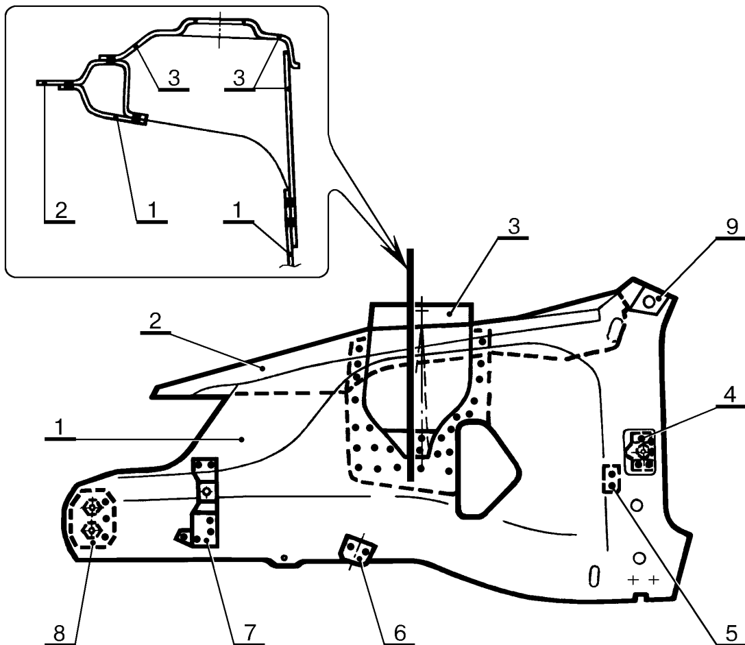
Рис.15. Детали брызговика переднего крыла в сборе (2110-8403260/261) правого/левого. Номера и наименования деталей, количество и шаг сварочных точек приведены в таблице 15 (всего 90±1/93±1 точка).
