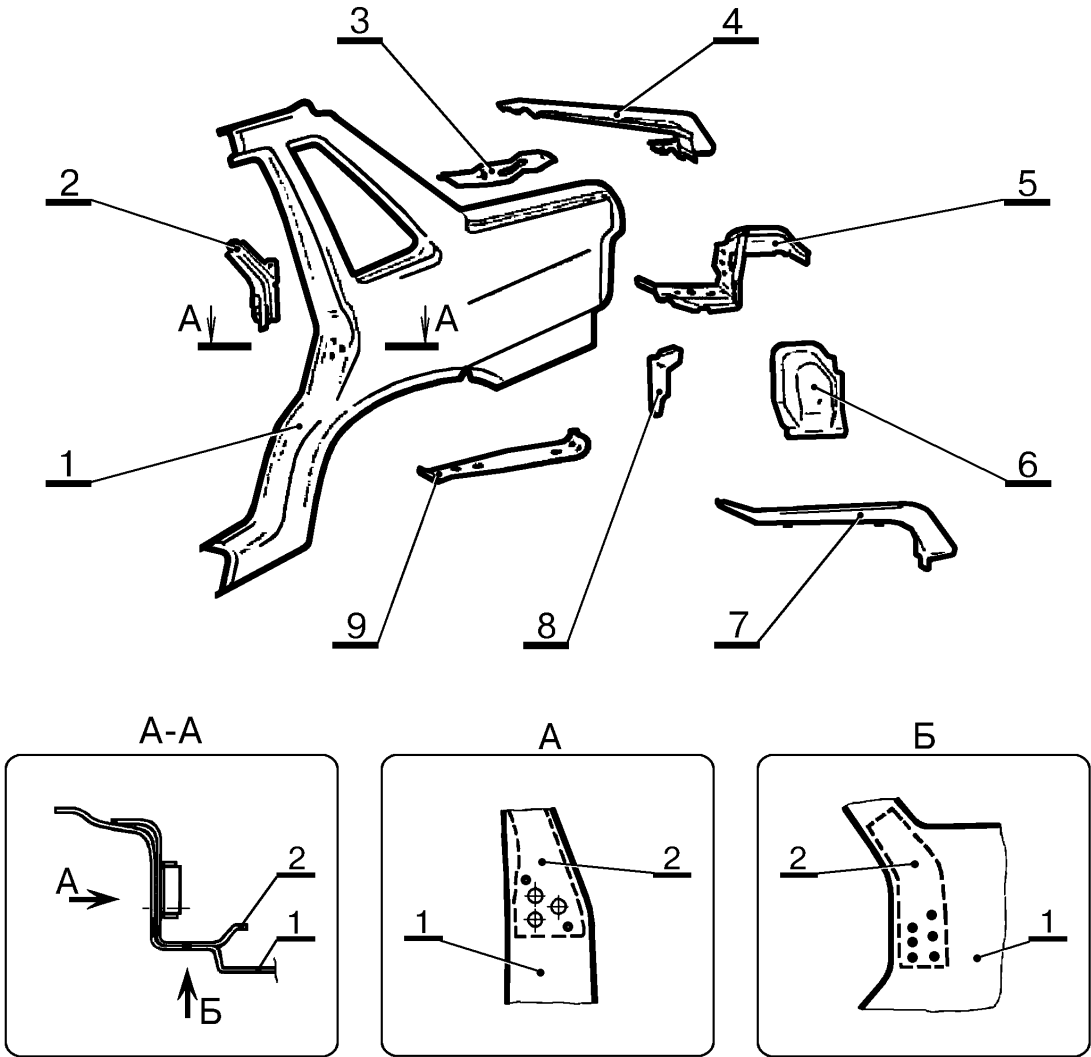
Рис.7. Детали крыла ВАЗ-21099; 2115 заднего в сборе правого/левого. Номера и наименования деталей, количество сварочных точек приведены в таблице 7.
