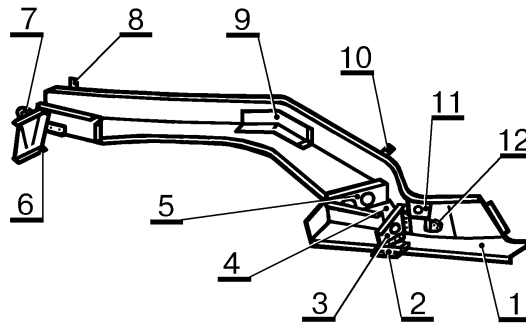
Рис.15. Детали лонжерона пола 2108; 21099-5101372/373 заднего в сборе. Номера и наименования деталей, количество сварочных точек приведены в таблице 15.
