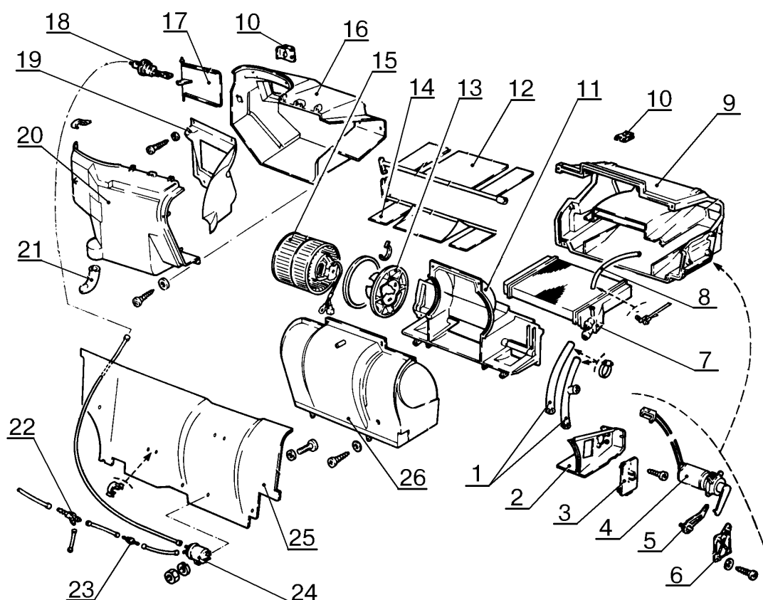
Рис.1. Детали отопителя.
