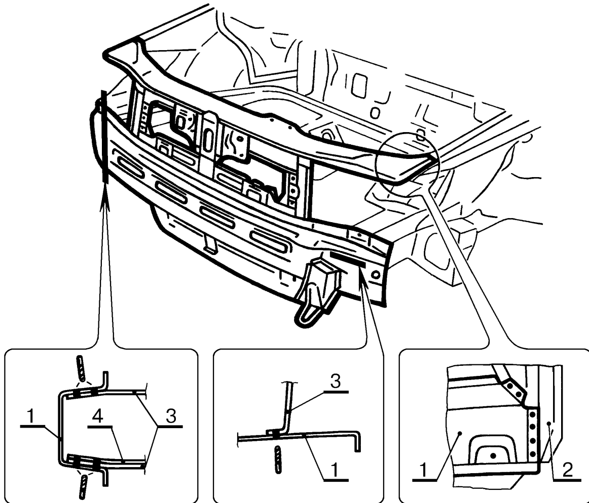
Рис.12. Соединение рамки радиатора в сборе с сопрягаемыми деталями. Количество и шаг сварочных точек по таблице 12.
