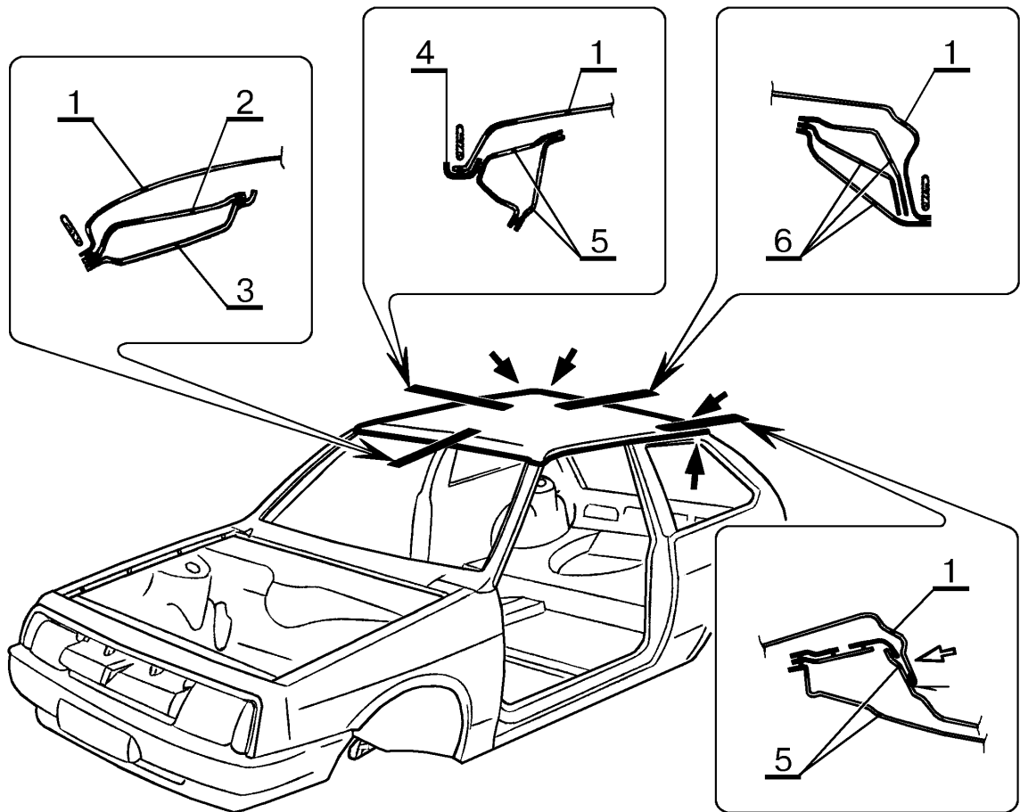
Рис.12. Соединение панели крыши ВАЗ-2108; 2109; 21099; 2114; 2115 с сопрягаемыми деталями (при снятых дверях). Места, указанные стрелками, проварить сплошным швом, аналогично заводским (см. поз.5 табл.12).
