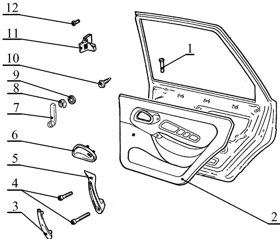
Рис.4. Обивка двери.
