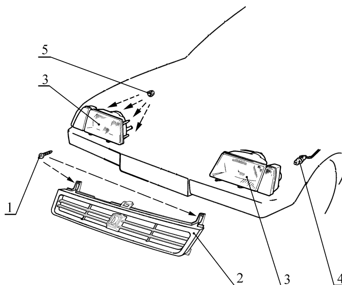
Рис.1. Блок-фары 2108-3711010/011:
