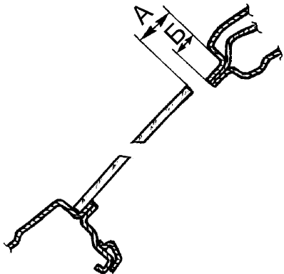
Рис.5. Проем ветрового стекла.
