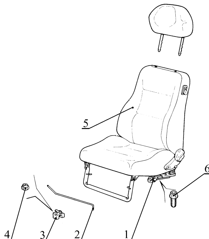
Рис.1. Сиденье переднее:
