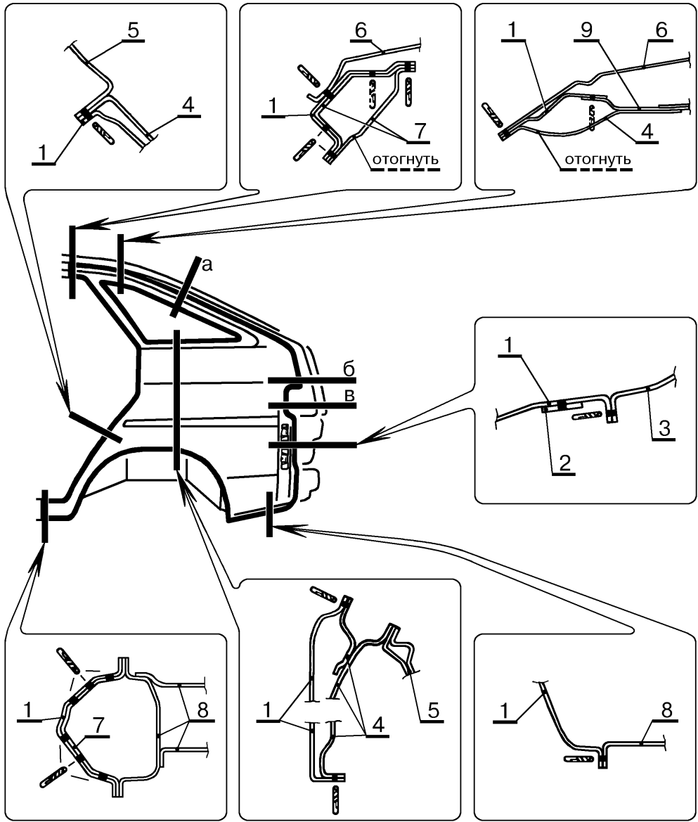
Рис.24. Соединение крыла заднего ВАЗ-2112 правого или левого с сопрягаемыми деталями (при снятой двери задка). Количество сварочных точек по таблице 24.
