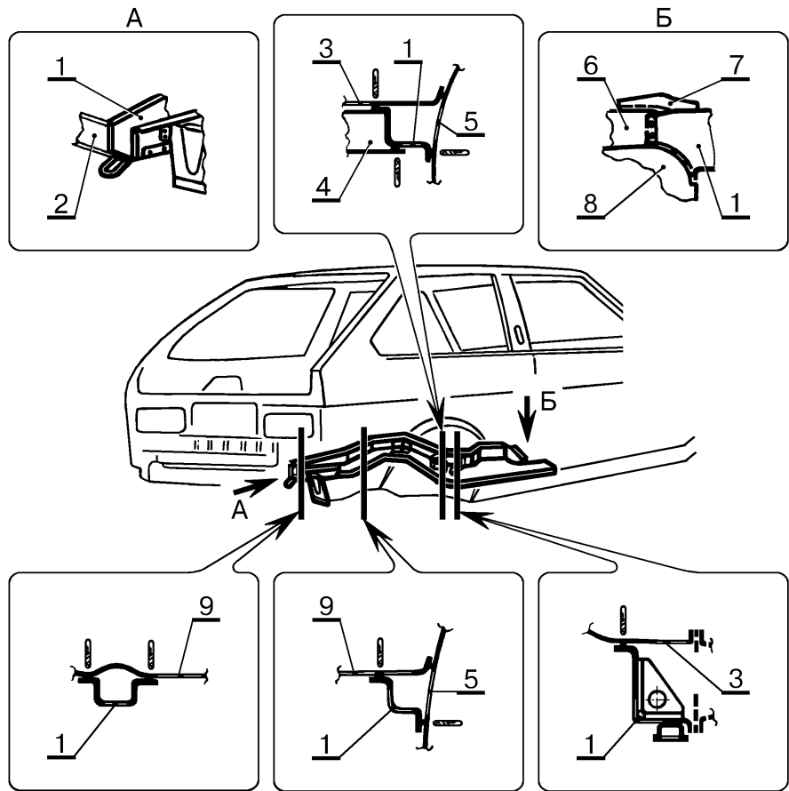
Рис.14. Соединение лонжерона пола 2108; 21099-5101372/373 заднего в сборе правой или левой с сопрягаемыми деталями (при снятых панели боковины в сборе правой или левой и панели задка).
