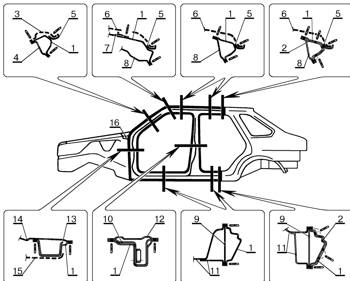
Рис.6. Соединение боковины кузова 21099; 2115-5401060/061 правой или левой с сопрягаемыми деталями (при снятых переднем крыле правом/левым, панели крыши и панели рамы ветрового окна).
