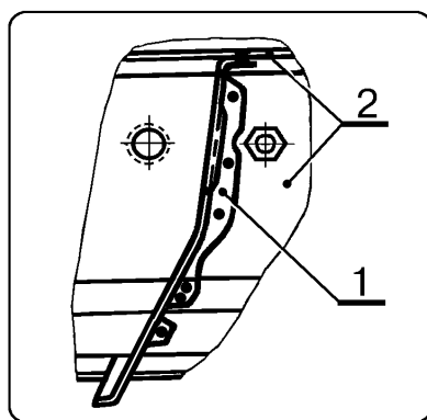
Рис.11. Соединение стойки рамки радиатора в сборе правой/левой с сопрягаемыми деталями.
