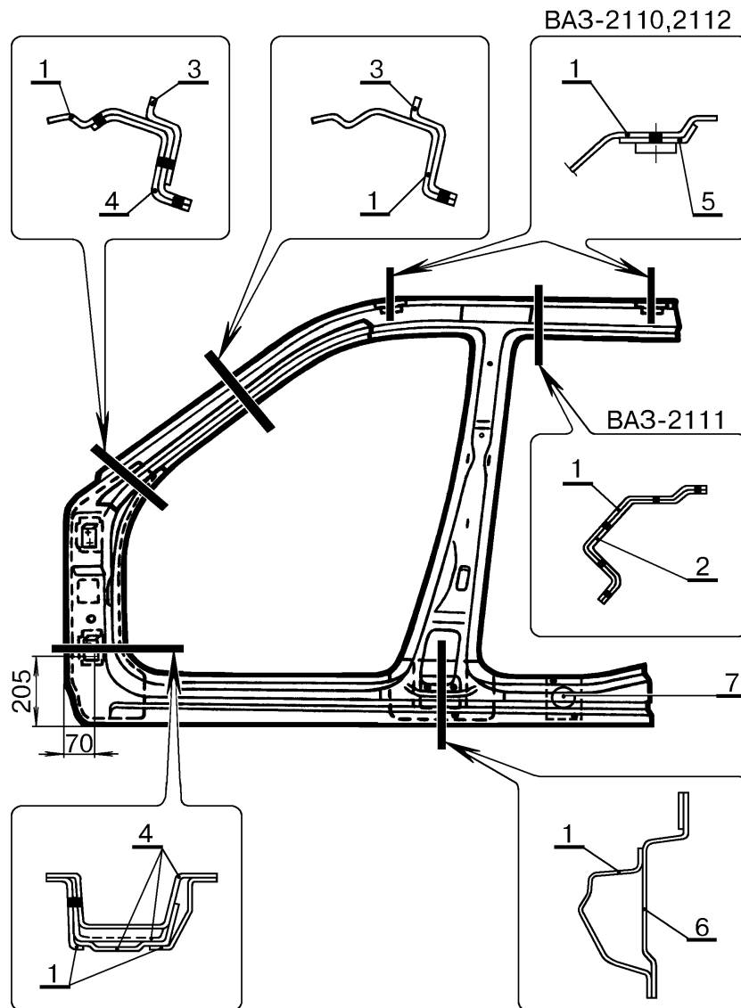
Рис.10. Детали боковины кузова в сборе правой или левой и надставка боковины верхняя (для ВАЗ-2111) правая или левая. Номера и наименования деталей, количество и шаг сварочных точек приведены в таблице 10 (всего для ВАЗ-2110; 2112 58/58 точек, для ВАЗ-2111 52 + 5/52 + 5 точек).
