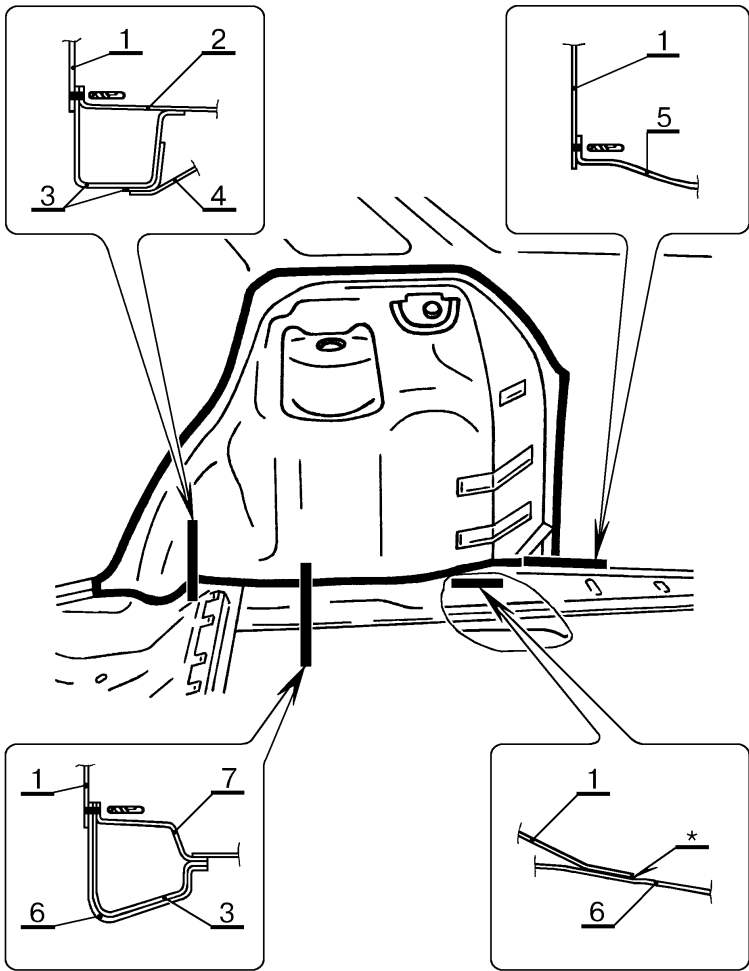
Рис.4. Соединение арки заднего колеса внутренней в сборе правой или левой с сопрягаемыми деталями (при снятой крышке багажника или двери задка, желобке заднего крыла, заднем крыле, панели задка угловой наружной (для ВАЗ-2110), арке заднего колеса наружной с угловой панелью боковины в сборе).
