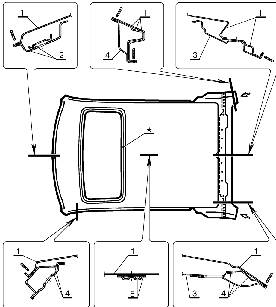
Рис.5. Соединение панели крыши в сборе ВАЗ-2112 с сопрягаемыми деталями (при снятых дверях). Места, указанные стрелками, проварить сплошным швом длиной 50 мм (см. поз.4 табл.5)
