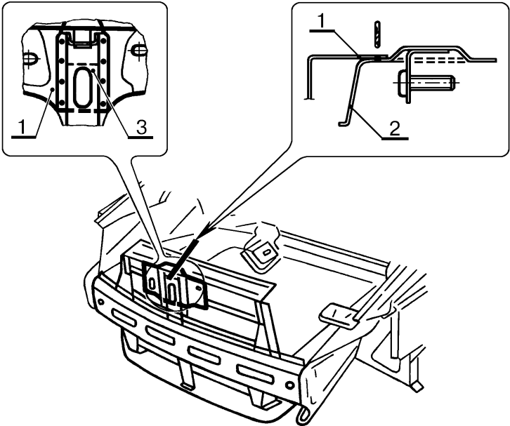
Рис.5. Соединение усилителя панели рамки радиатора в сборе с сопрягаемыми деталями
