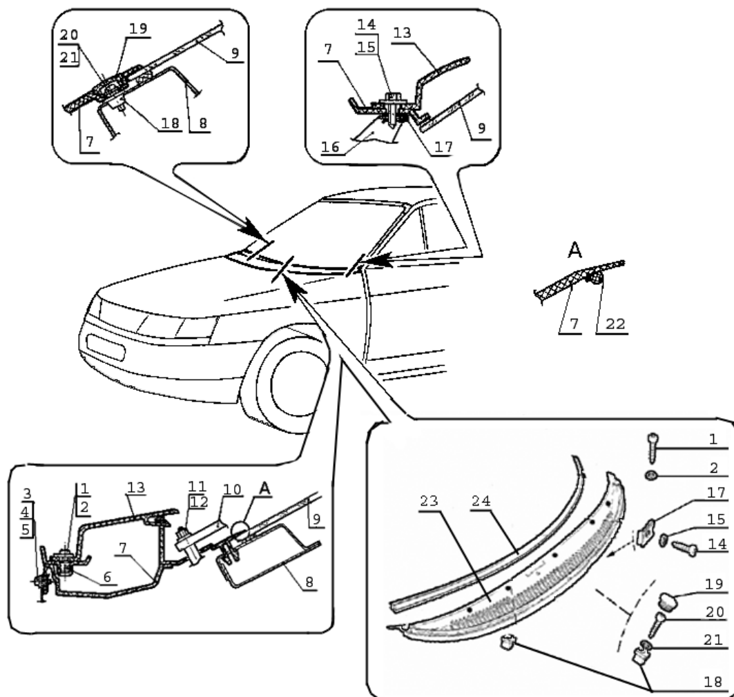
Рис. 2. Установка накладки и облицовки рамы ветрового окна:
