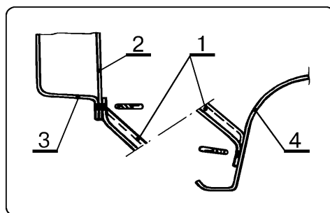
Рис.10. Соединение усилителя панели облицовки радиатора нижнего с сопрягаемыми деталями.
