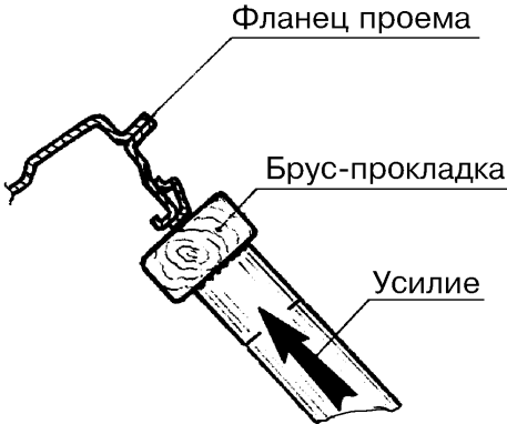
Рис.6. Правка проема.
