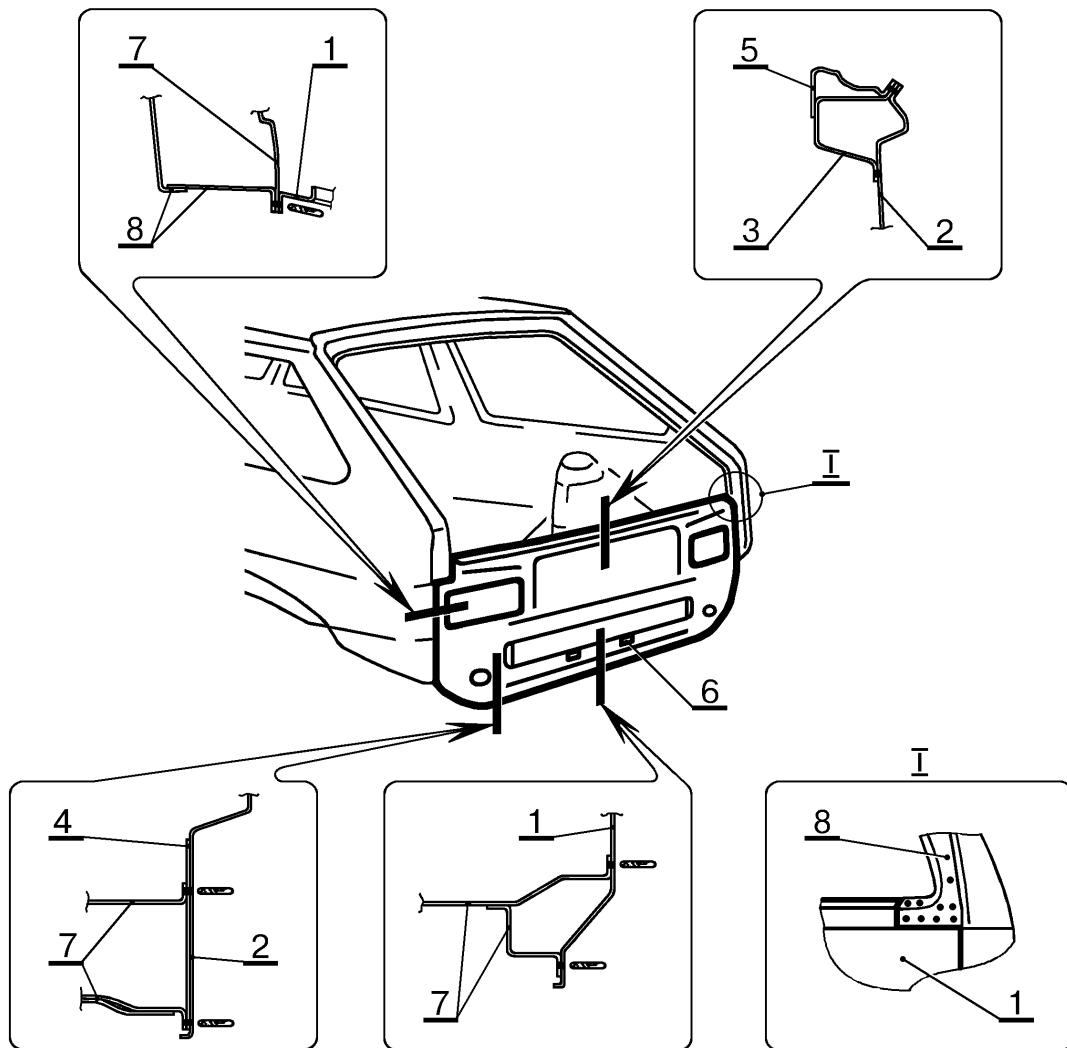
Рис.10. Соединение панели 2108-5601080 задка в сборе с сопрягаемыми деталями.
