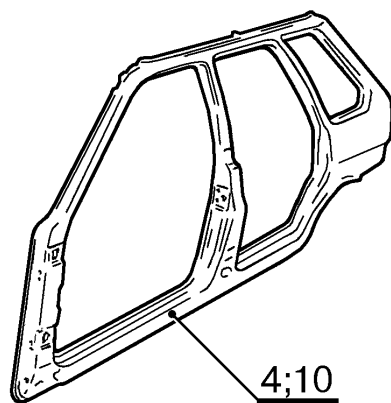
Рис.1. Детали средней части кузова ВАЗ-2108; 2109; 21099; 2114; 2115. Номера деталей, наименования и применяемость приведены в таблице 1.
