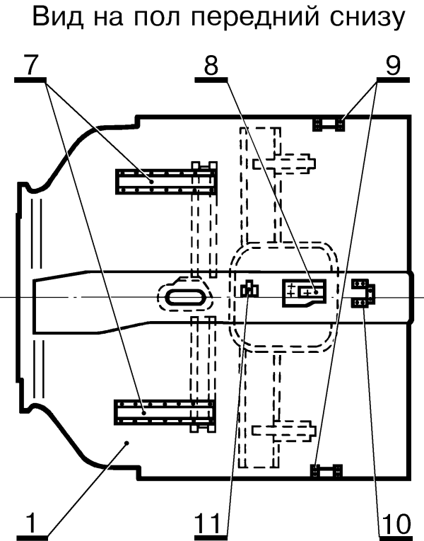
Рис.12. Детали пола переднего в сборе. Номера и наименования деталей, количество и шаг сварочных точек приведены в таблице 12 (всего 175 \pm 1 точка).
