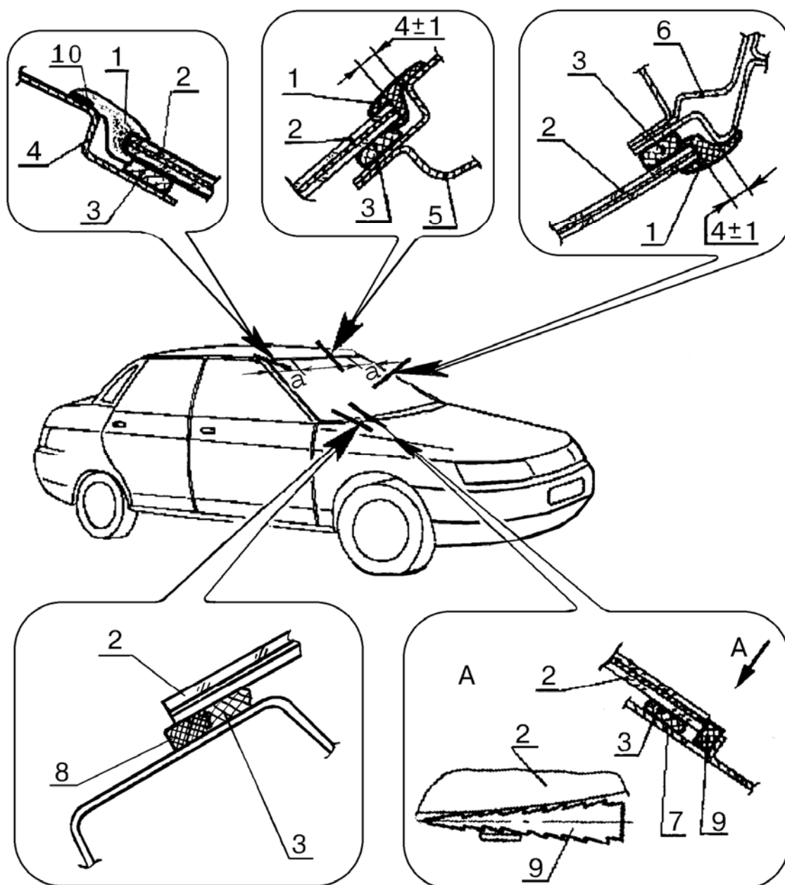
Рис. 4. Установка стекла и окантовок ветрового стекла:
