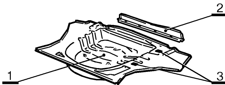
Рис.3. Детали пола заднего в сборе ВАЗ-2108; 2109; 2114. Номера и наименования деталей, количество сварочных точек приведены в таблице 3.
