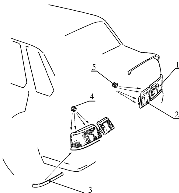
Рис.2. Фонари задние а/м ВАЗ-2115:
