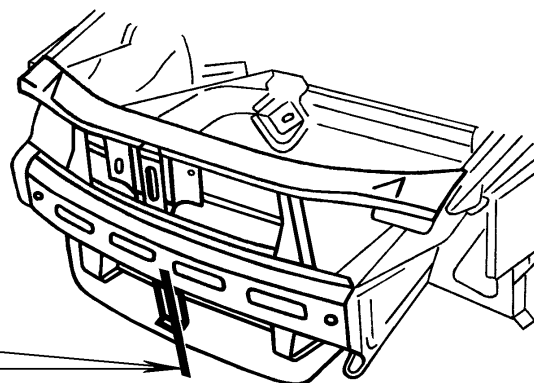
Рис.10. Соединение усилителя панели облицовки радиатора нижнего с сопрягаемыми деталями.
