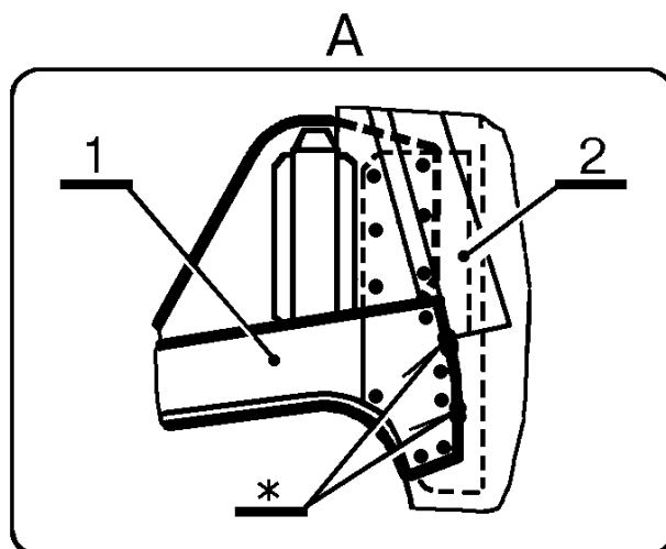
Рис.8. Соединение поперечины рамы ВАЗ-21099; 2115 заднего окна нижней в сборе с сопрягаемыми деталями (при снятой крышке багажника).
