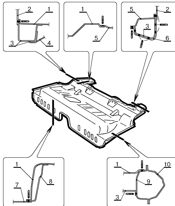
Рис.13. Соединение пола среднего в сборе, рис.14, с сопрягаемыми деталями (при снятом капоте, передних и задних дверях, крышке багажника и задних крыльях).
